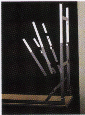
脚部の長さ調節・折りたたみ
