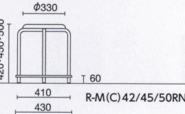
R-C42RN ¥18,100 質量:2.6kg 仕様:φ22.2メッキ脚 スタッキング6脚 4
