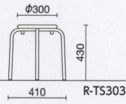
R-TS303 ¥16,400 質量:2.7kg 4
