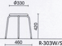
R-303W ¥9,700 質量:1.8kg 仕様:φ22.2ホワイト塗装脚 スタッキング6脚 6
